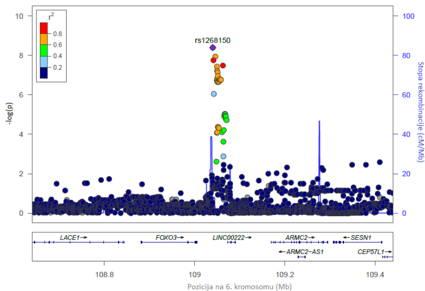
Slika 11. Dijagram povezanosti pripadne genomske regije za polimorfizam rs1268150.
