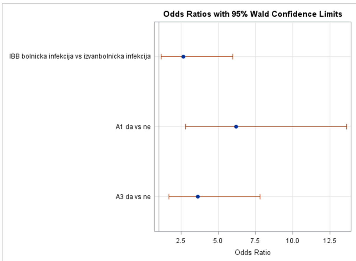
Slika 4. Omjeri izgleda sa 95%-tnim intervalima pouzdanosti za prediktore u multivarijantnom modelu (2) logističke regresije.
