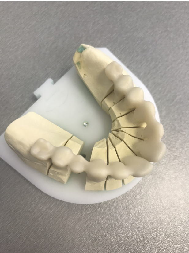
Slika 3. Cirkonij-oksidne jezgre za most (ljubaznošću izv. prof. dr. sc. Tee Galić, dr. med. dent.)
