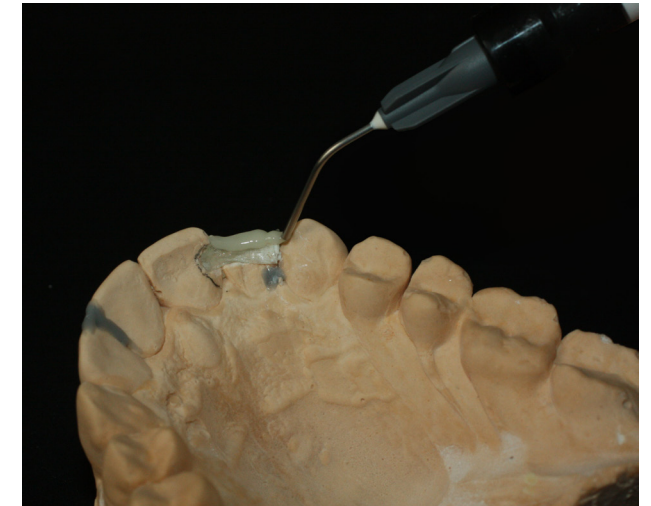
Slika 4. Staklena vlakna postavljena su kao potpora kompozitu.
