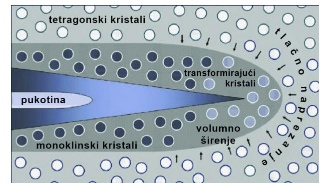
Slika 2. Transformacijsko ojačanje (Preuzeto i modificirano prema 5)
